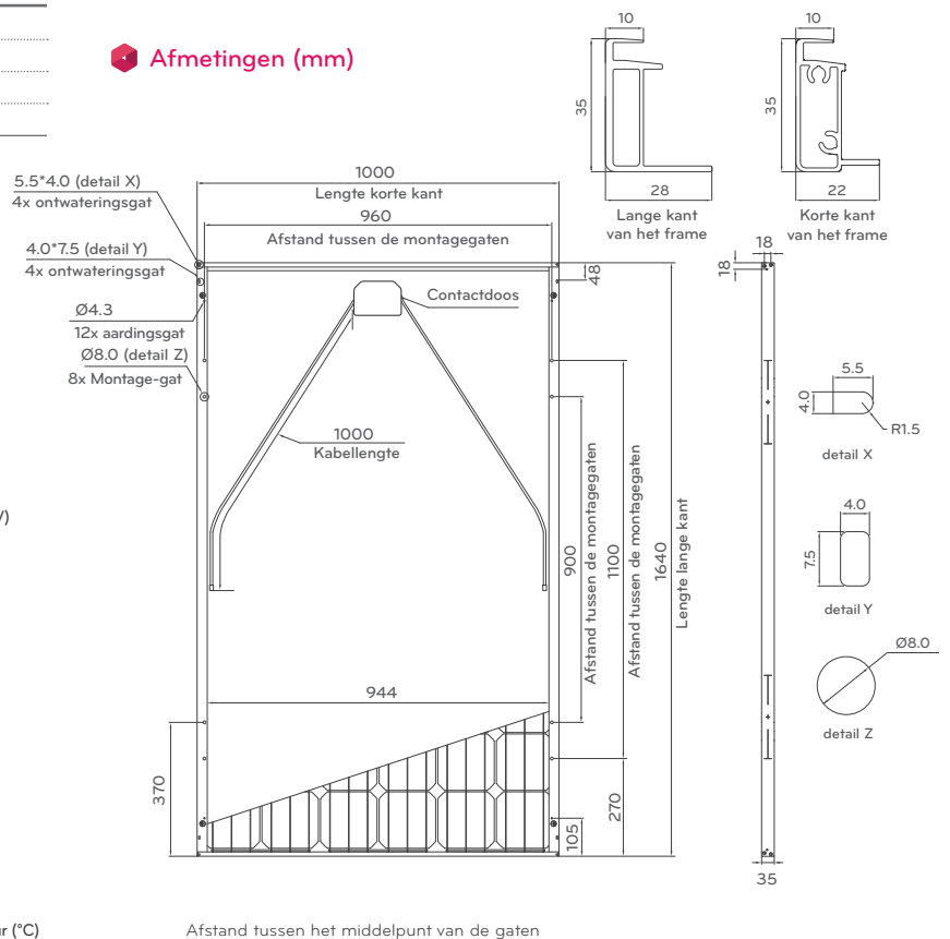
Afstand tussen het middelpunt van de gaten
